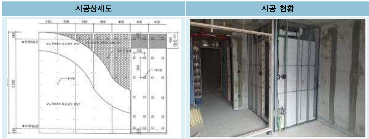
[그림 8] 시공상세도 및 현장 시공현황
